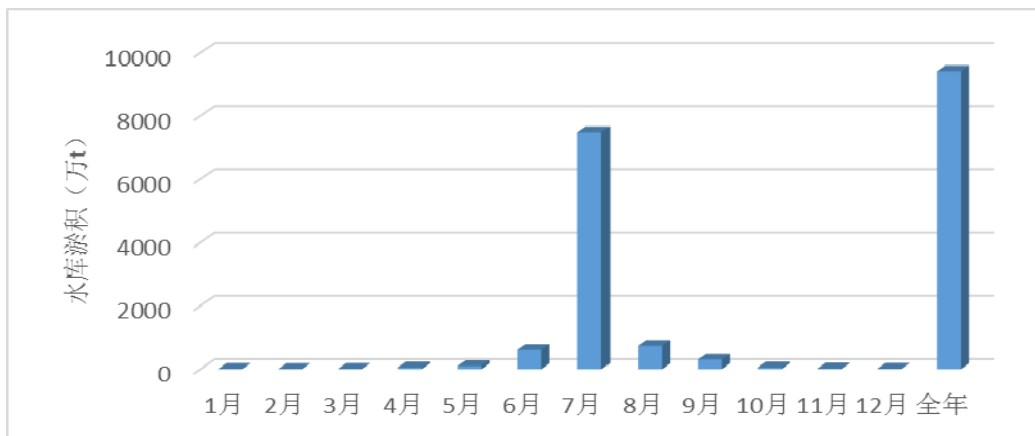
图 5-3 三峡水库库区 2013 年逐月淤积量变化
