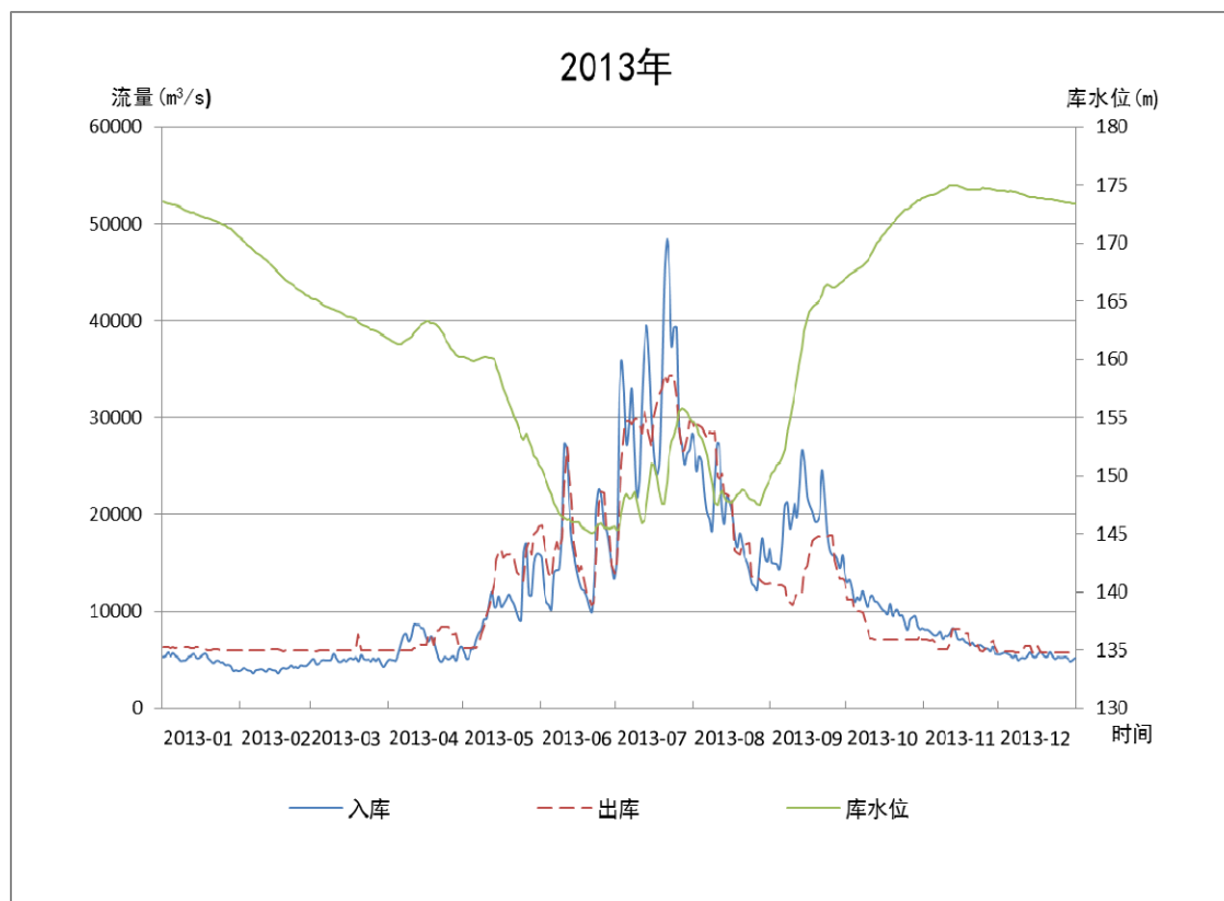
图 2-1 2013 年三峡水库库水位及出入库流量过程线
