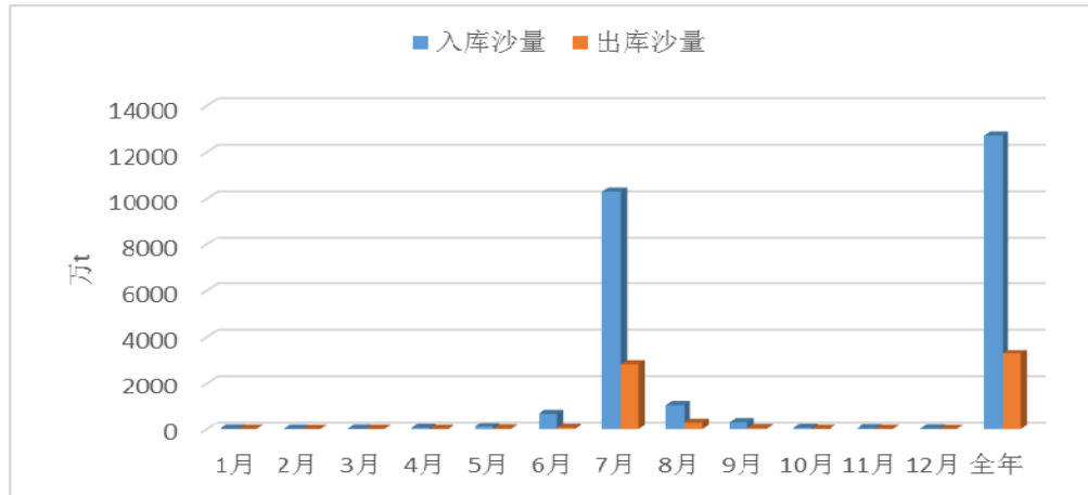
图 5-2 三峡水库 2013 年逐月出入库沙量
